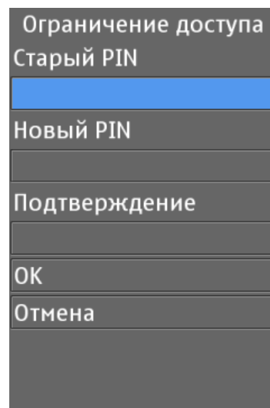
Рис. 9: Смена PIN-кода
