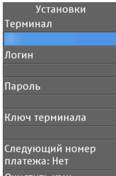
Рис. 1: Установки
