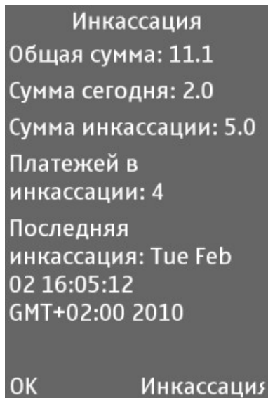
Рис. 7: Инкассация
