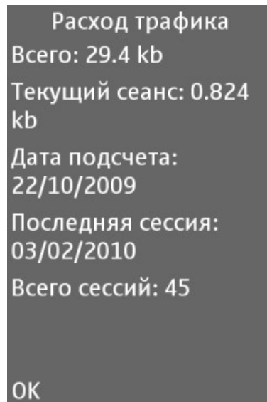
Рис. 8: Расход трафика
